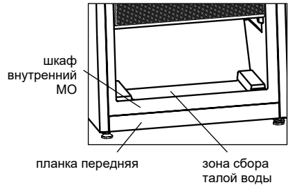
Рисунок 10 – Сбор талой воды из МО
