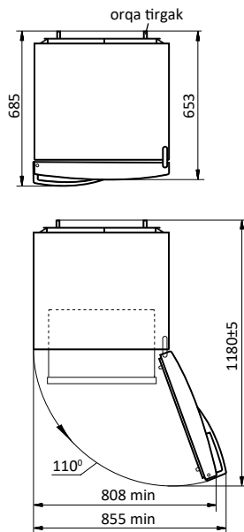
2-rasm – Sovutgich (yuqoridan ko'rish)
